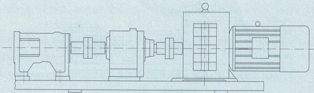
齿轮配合电磁调速电机驱动
